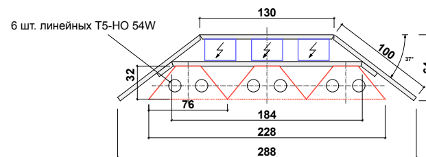
Поперечный разрез.
