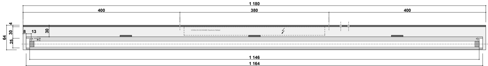
Продольный разрез.
